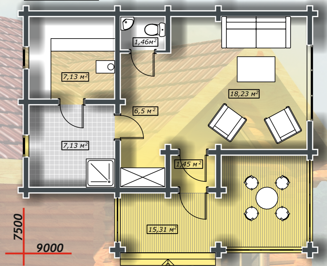
План бани
