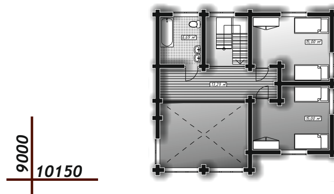
План 2 этажа
